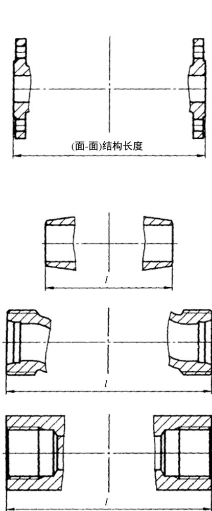
图 1 直通式阀门结构长度
